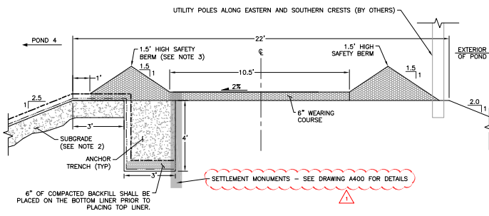
E E TYPICAL POND CREST A110 A115
